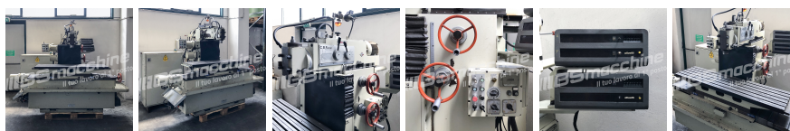
Fresatrice fresa verticale usata C.B. FERRARI P4R motorizzata e visualizzata 3 assi.
